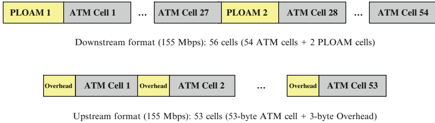
Fig. 2.2 APON frame format
